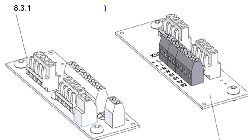
Scheda di connessione Circuito di monitoraggio
